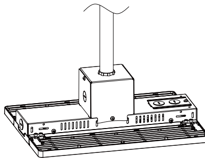
Pendant Mount
