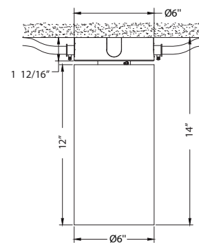
Conduit Surface Mount
