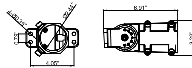
MSF-AR-G2 ( \pm 35^\circ )
