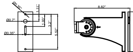
MAM-AR-G2 ( \pm 90^\circ )
